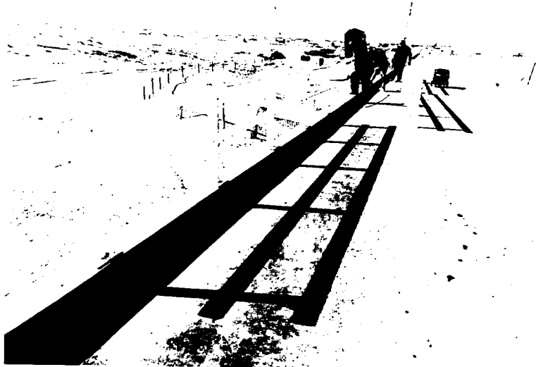
FOTO 11: Instalación de barandas en el sardinel del muelle San José
