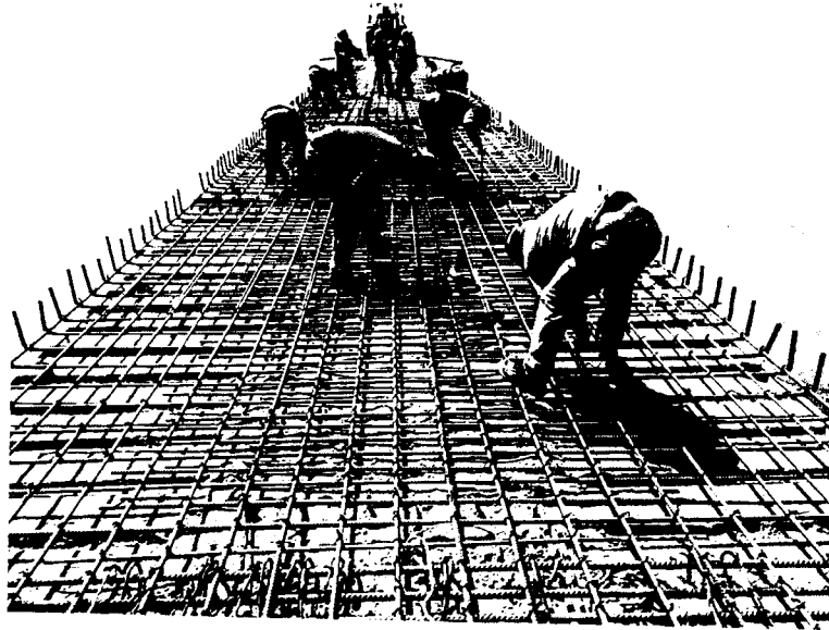
FOTO 01: Armado de acero en losa del día 01/07/19
